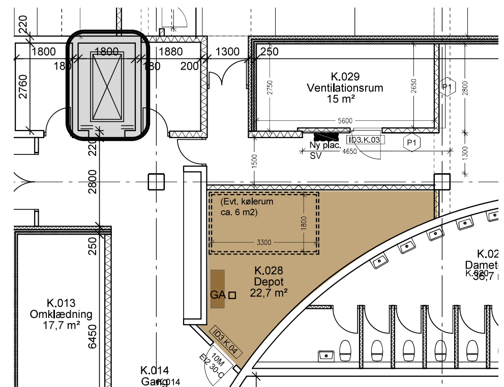
Plan kælder
